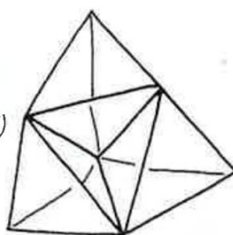
Ottaedro stellato (12 moduli)
