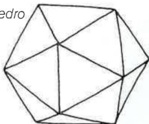
Icosaedro stellato (30 moduli)
