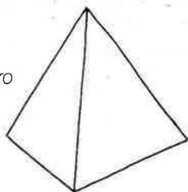
Tetraedro stellato (6 moduli)
